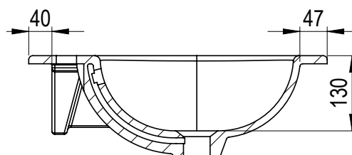
SEZIONE A-A
