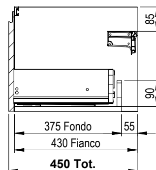
SEZIONE A-A
