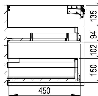
SEZIONE A-A
